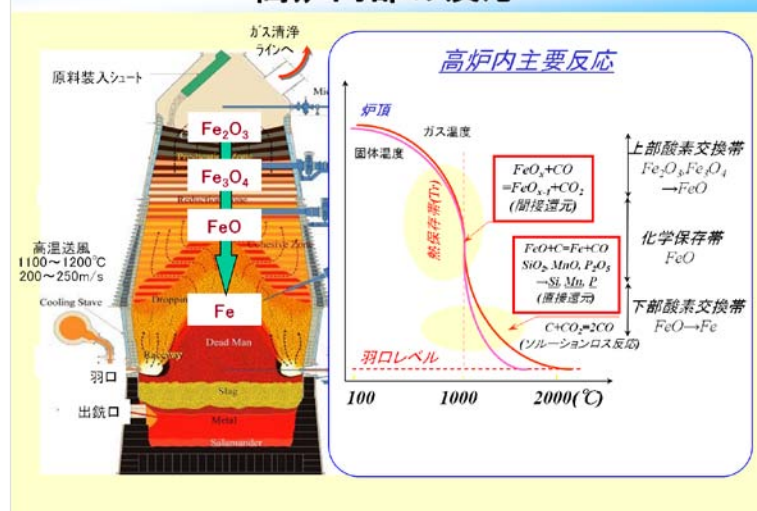
高炉内部の反応
